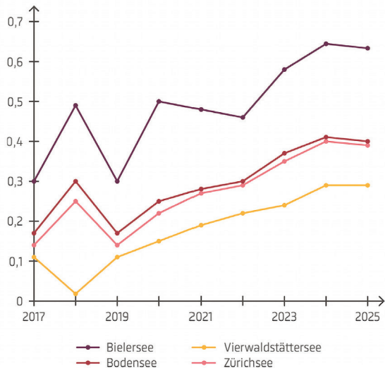
Abbildung 2: Trifluoressigsäure-Konzentrationen in vier Schweizer Seen von 2017 bis 2025. Proben wurden jeweils einmal pro Jahr im Frühjahr genommen. Quelle: AWBR (2025)
